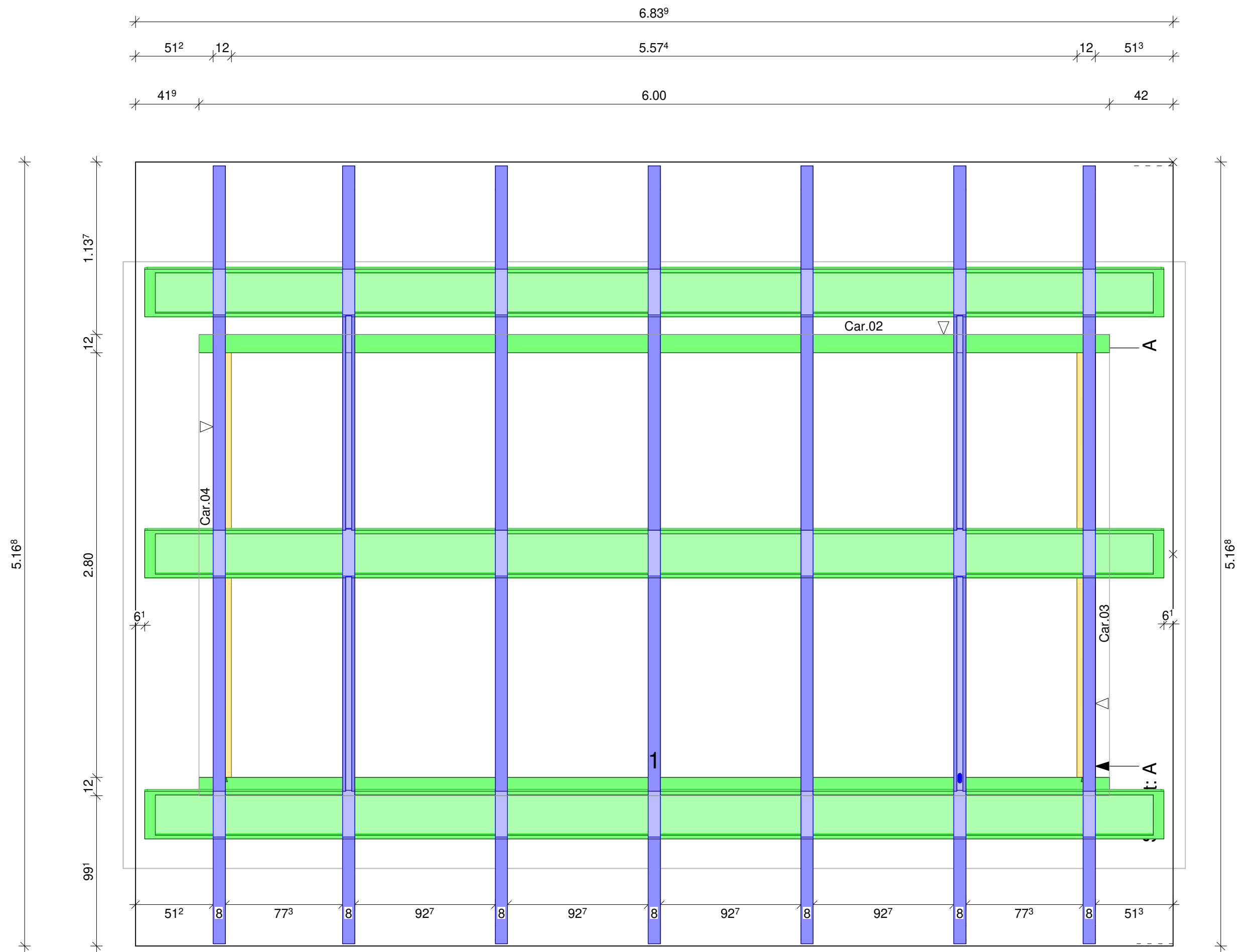
Solarcarport Typ III, 2 Stellplätze, 18 Module
